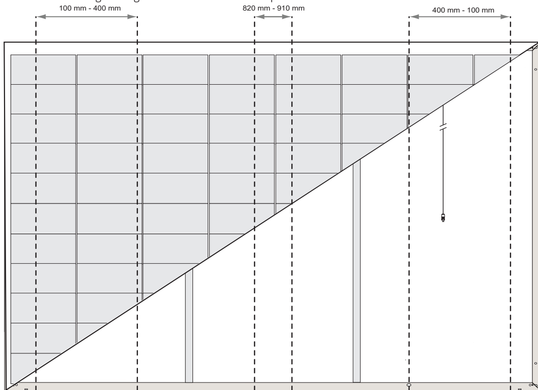
Abb. 5-4 Sechspunkt-Montage Konfiguration Klemmzonen: REC Alpha Pure-RX-Serie
