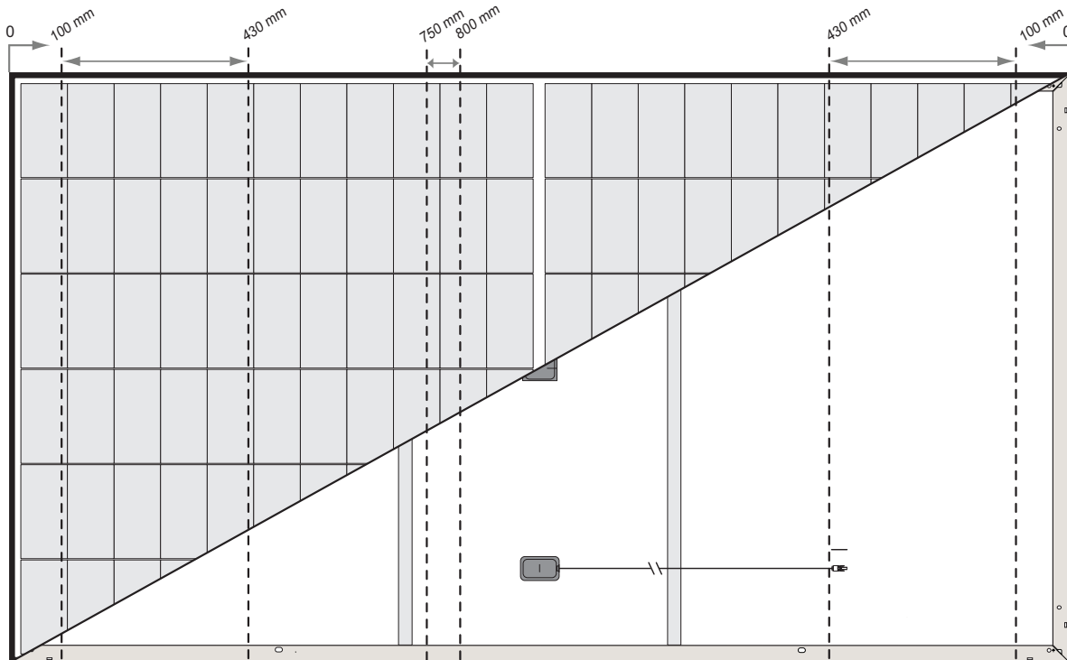
Abb. 3-4 Sechs-Punkt-Montage Konfiguration Klemmbereiche: REC Alpha Pure 2-Serie
