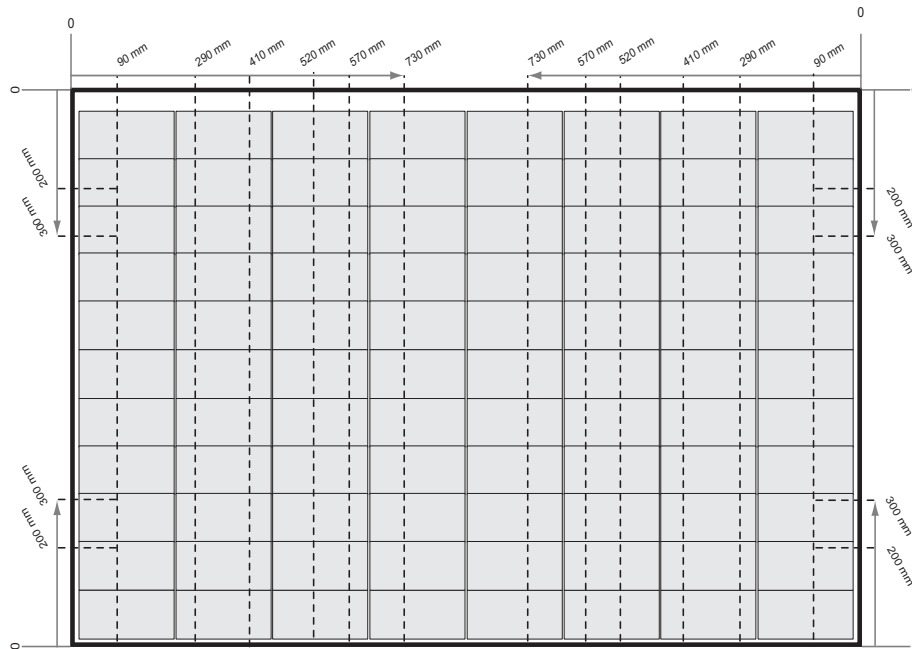
Abb. 5-1 Klemmung von Module der REC Alpha Pure-RX-Serie mit Schienen parallel zur kurzen Seite des Moduls
