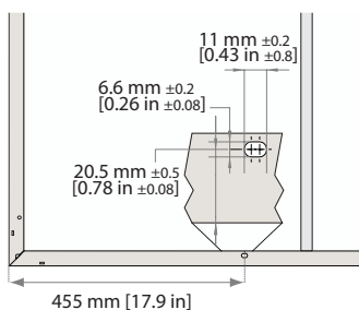
Abb. 3 Beispiel für die Montage von Befestigungslöchern
