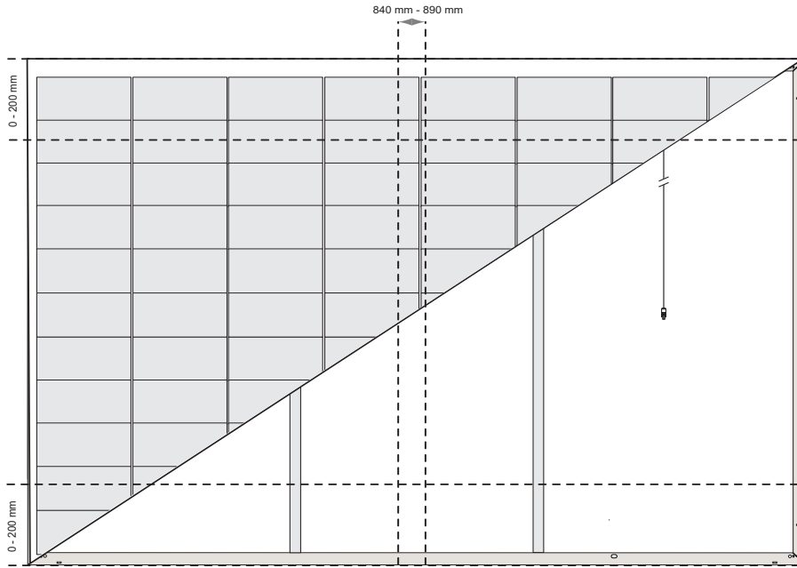
Abb. 5-5 Gemischte Sechs-Punkt-Montage von Module der REC Alpha Pure-RX-Serie mit kurzen Schienen
