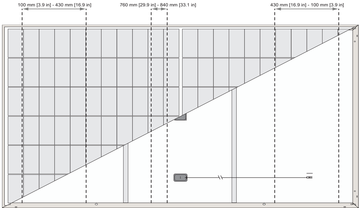
Abb. 2-4 Sechsstück-Montagekonfiguration Klemmbereiche: REC Alpha Pure-Serie
