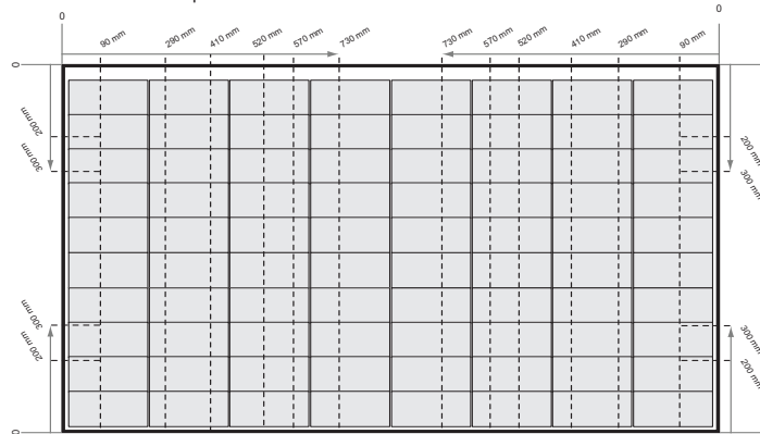
Abb. 4-3 Klemmen von Module der REC Alpha Pure-R Serie mit kurzen Schienen
