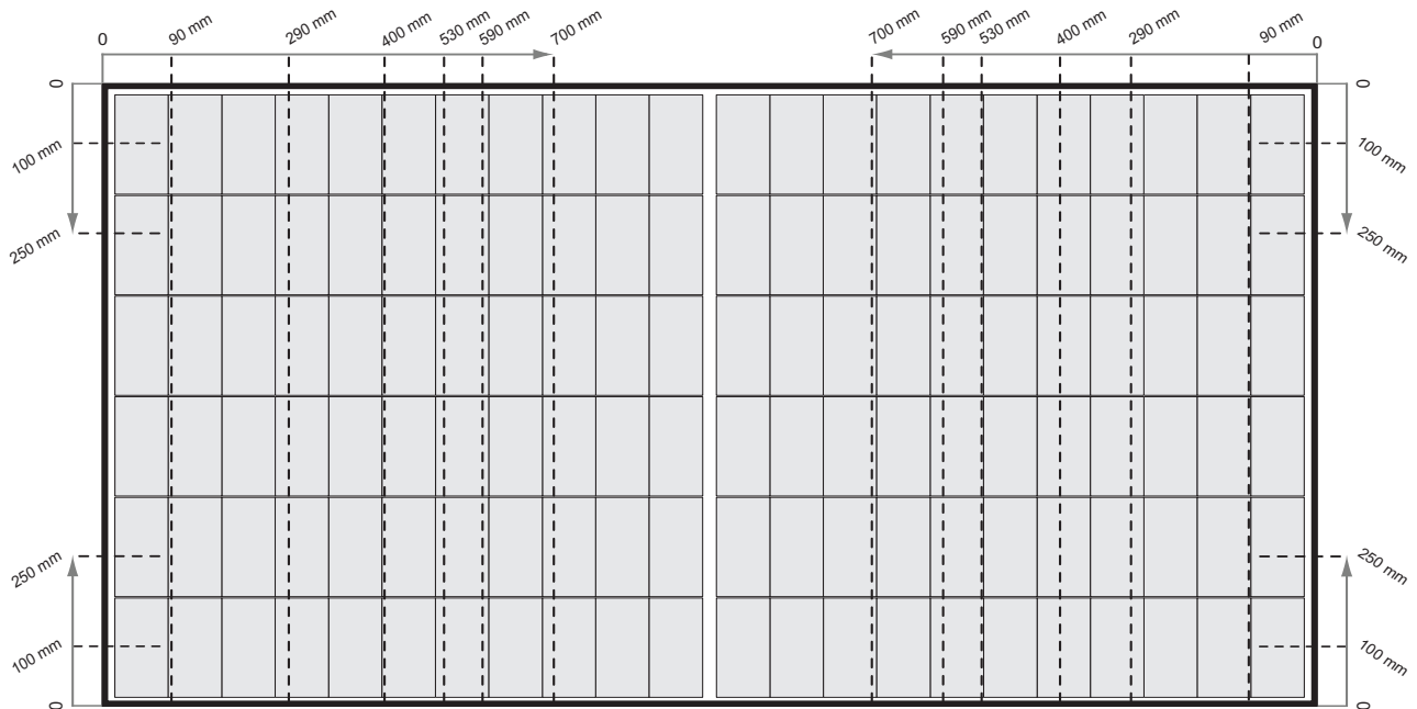
Abb. 3-1 Klemmung von REC Alpha Pure 2 Module mit Schienen parallel zur kurzen Seite des Moduls
