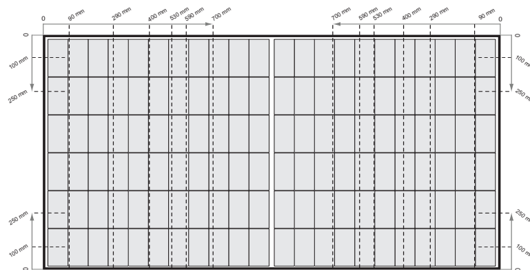
Abb. 3-3 Klemmung der REC Alpha Pure 2 Serie mit kurzen Schienen
