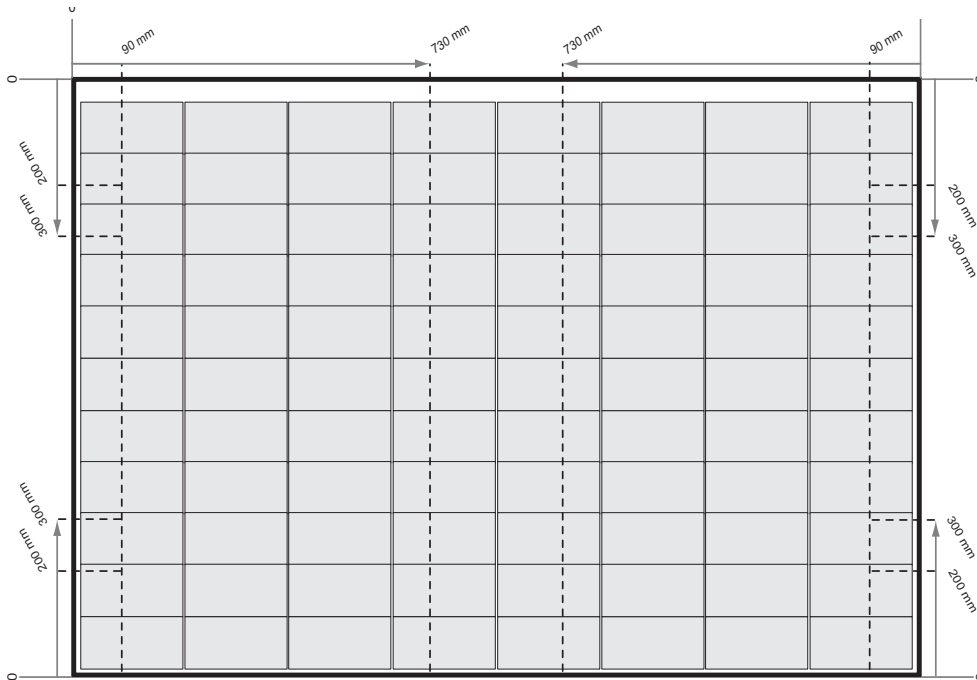
Abb. 5-2 Klemmung von REC Alpha Pure-RX Module mit Schienen parallel zur Längsseite des Moduls
