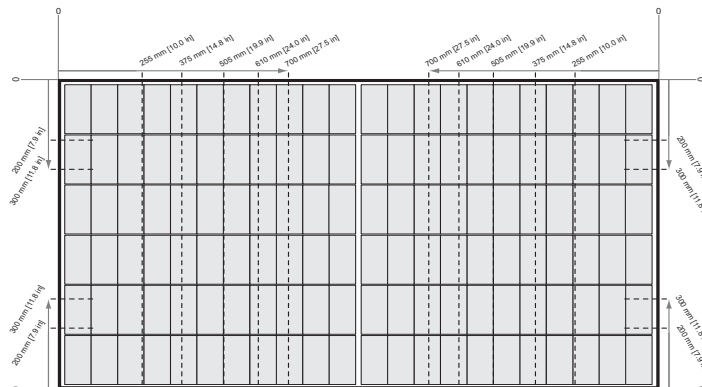
Abb. 2-3 Klemmung von Module der REC Alpha Pure-Serie mit kurzen Schienen
