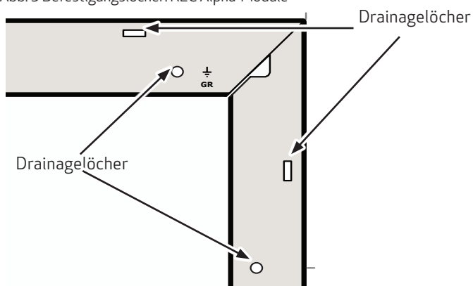
Abb. 5 Befestigungslöcher: REC Alpha-Module
