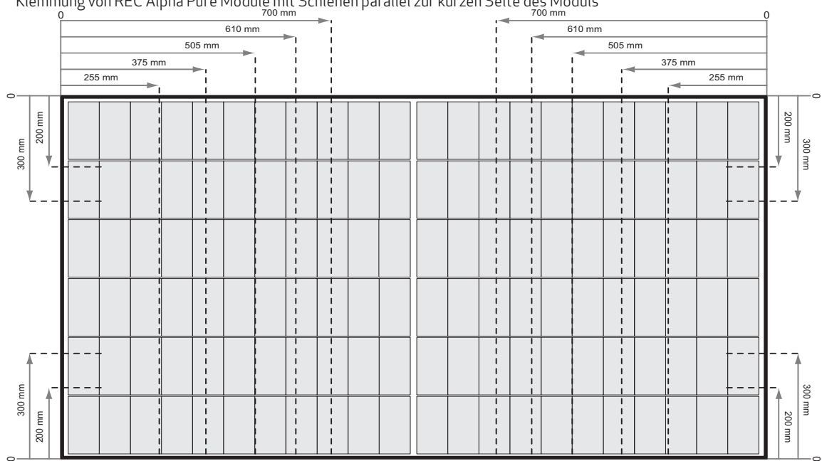
Abb. 2-1 Klemmung von REC Alpha Pure Module mit Schienen parallel zur kurzen Seite des Moduls
