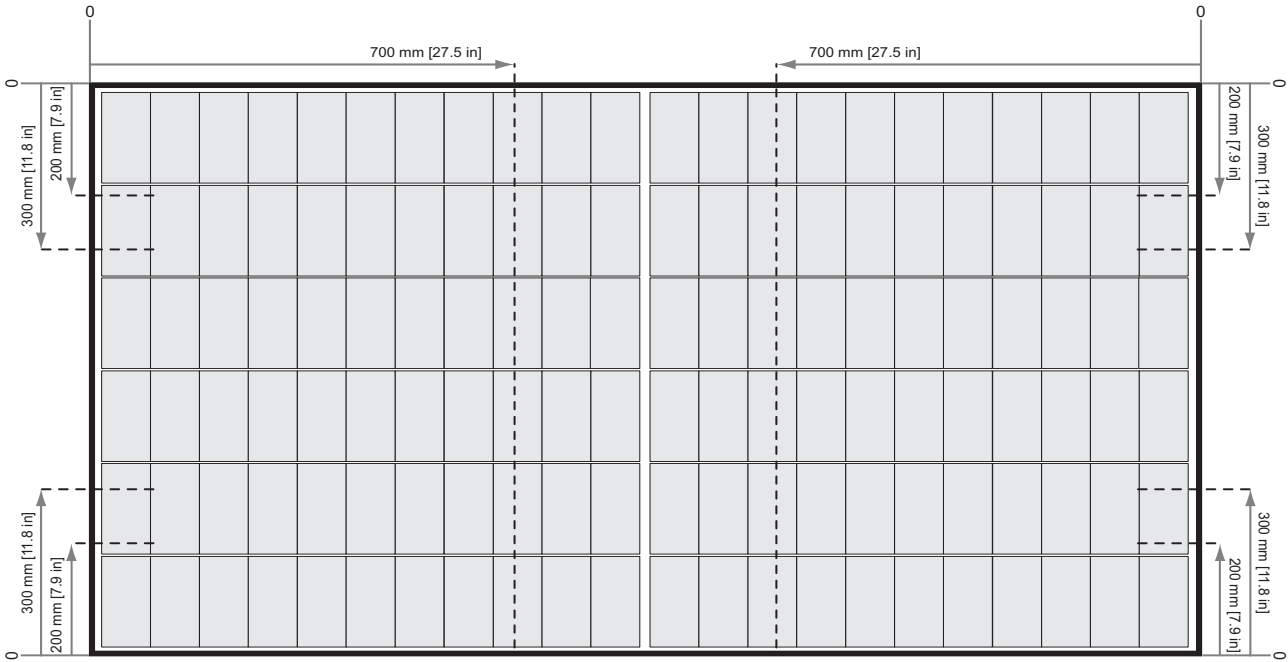
Abb. 2-2 Klemmung von Module der REC Alpha Pure Serie mit Schienen parallel zur Längsseite des Moduls
