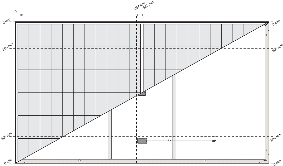
Abb. 3-5 Gemischte Sechs-Punkt-Montage von REC Alpha Pure 2-Modulen mit kurzen Schienen
