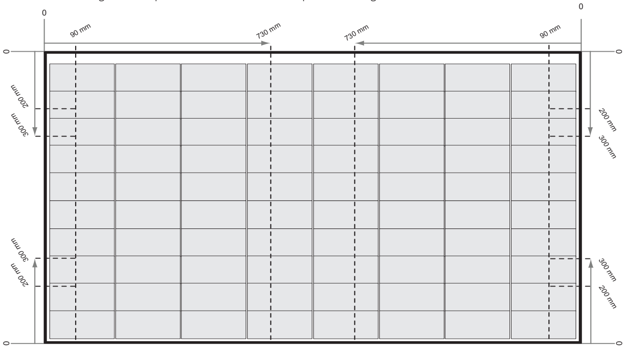
Abb. 4-2 Klemmung von REC Alpha Pure-R Module mit Schienen parallel zur Längsseite des Moduls
