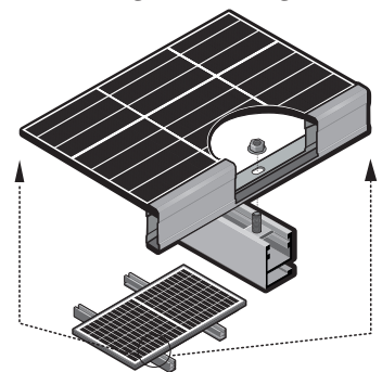
Abb. 4 Beispiel für die Montage eines Montagelochs
