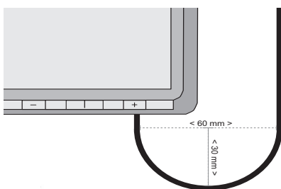
Abb. 6 Spezifikationen der Klemme
