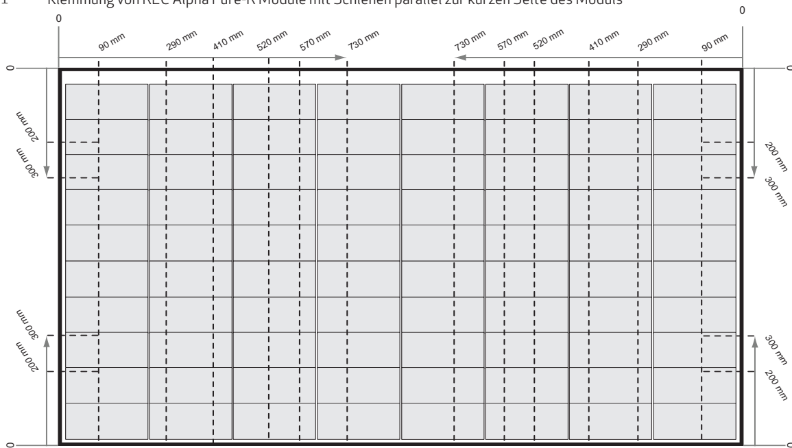
Abb. 4-1 Klemmung von REC Alpha Pure-R Module mit Schienen parallel zur kurzen Seite des Moduls
