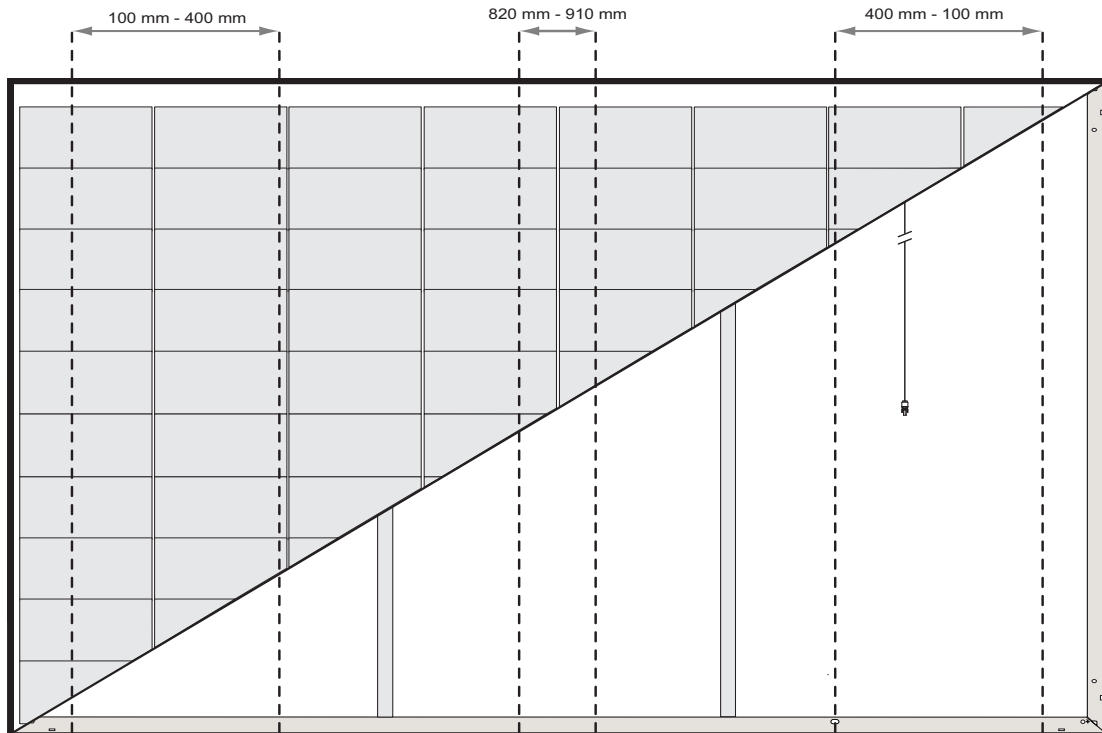
Abb. 4-4 Sechspunkt-Montagekonfiguration Klemmbereiche: REC Alpha Pure-R Serie
