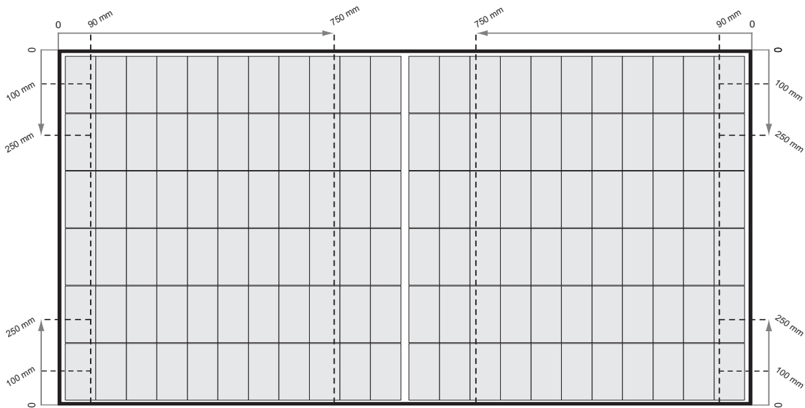
Abb. 3-2 Klemmung von REC Alpha Pure 2 Module mit Schienen parallel zur Längsseite des Moduls
